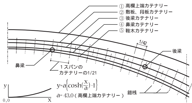
図-6 錦帯橋の基準カテナリーモデル図
