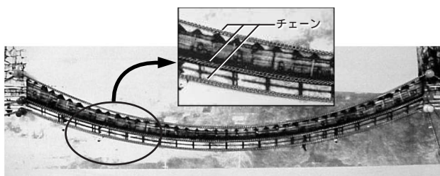
写真-2 1953年の錦帯橋の写真とカテナリー
